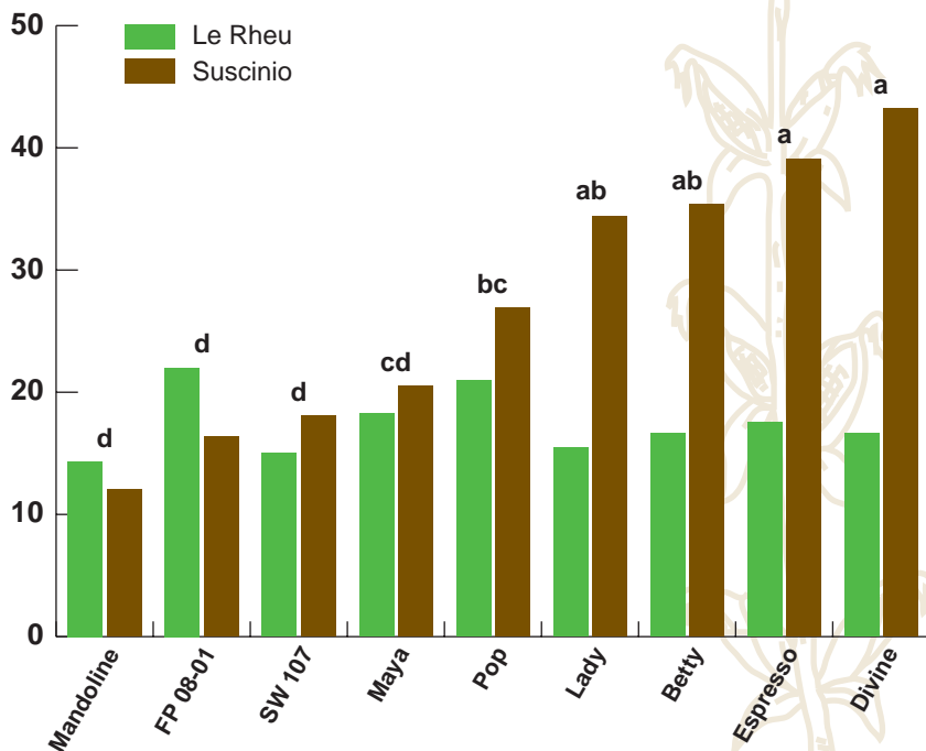
Figure 1 : Rendement par variété en fonction du lieu de production (en Q/ha) (et groupes homogènes pour le site de Suscinio)
